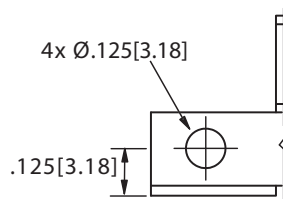
FLUSH with CLEARANCE HOLES (D)
