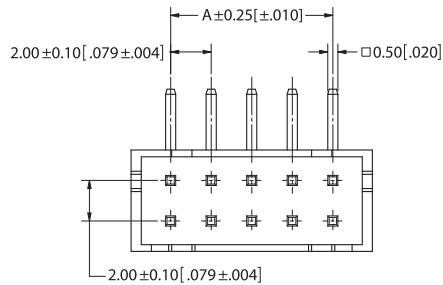
SWR204-NRTN-D__-RA-GA
