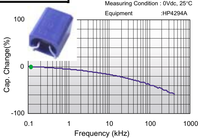
Organic 3628/47uF/10V
