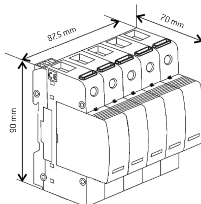
5 Poles
