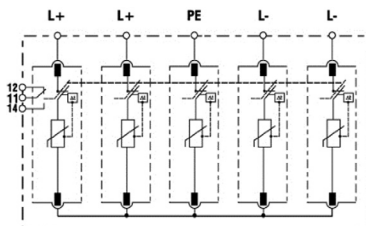
5 Poles
